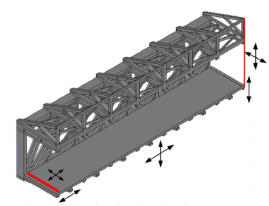
図-2 1/4 モデル
