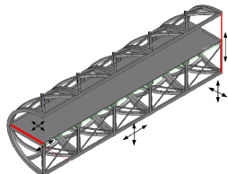
図-6 1/4 モデル
