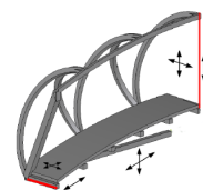
図-4 1/4 モデル
