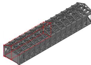
図-1 阿蘇望橋モデル あそぼうばし
