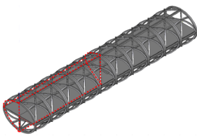
図-5 楕円断面モデル
